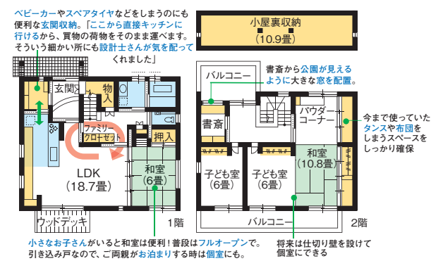
スタッフと細かい打ち合わせを重ねた間取りプラン
